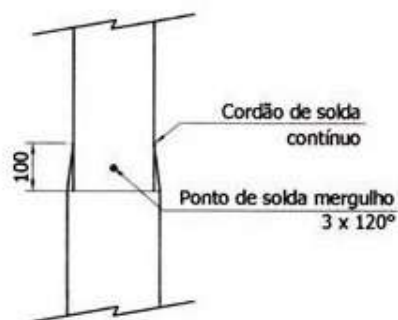
Detalhe 01
