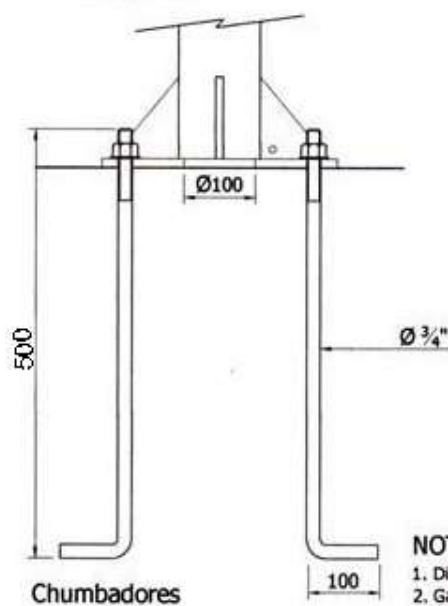
Detalhe 01
