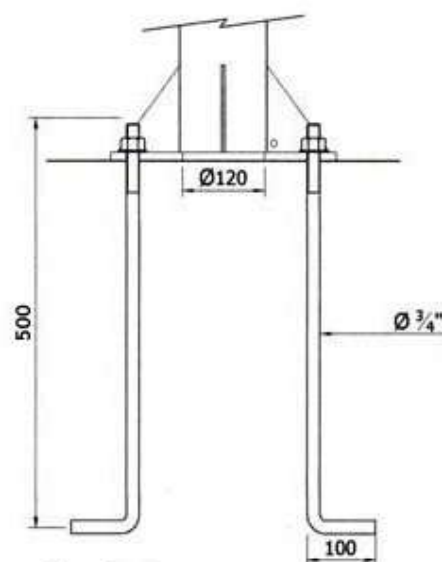
Chumbadores
