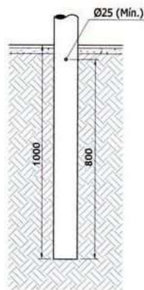
Detalhe do Engaste
