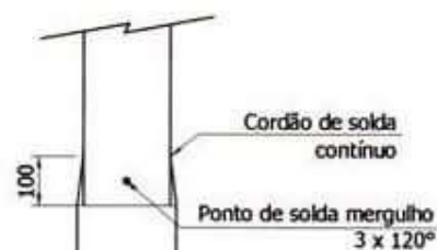
Detalhe 01a
