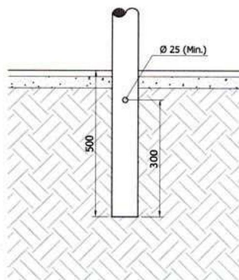
Detalhe de Engaste
