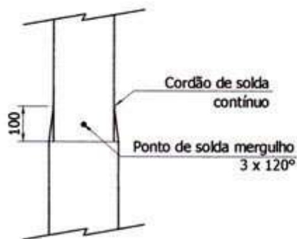
Detalhe 01
