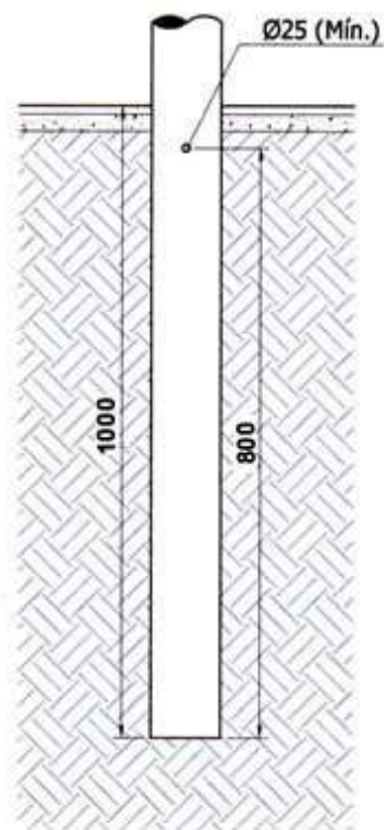
Detalhe do Engaste
